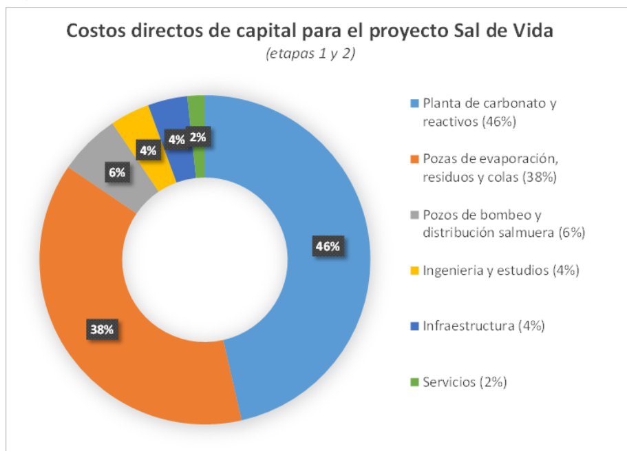
Figura 9: Estimación de costos de construcción para el proyecto Sal de Vida.
